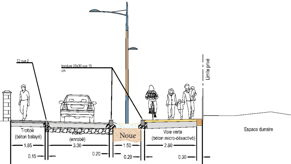
Profil type du boulevard Maritime de la rue des Chaumette à la rue de la Corderie
